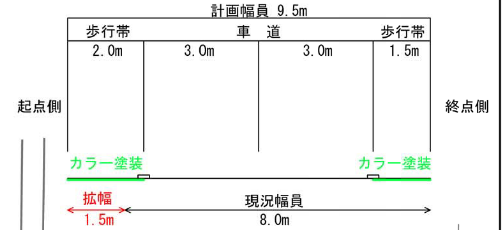
A-A' 断面図
