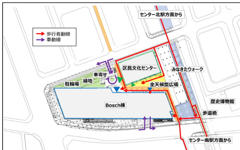
全体配置図
